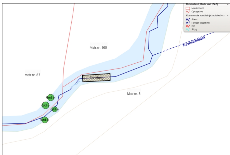
Figur 3. Placering af projektiltag 1 etablering af sandfang i ca. st. 430-440 m og projektiltag 2 plantning af rød-el i ca. st. 470-485 m.
