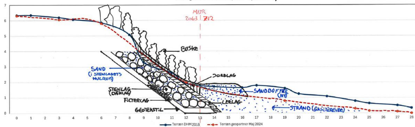
Figur 4 Tværnsit gennem anlægget
