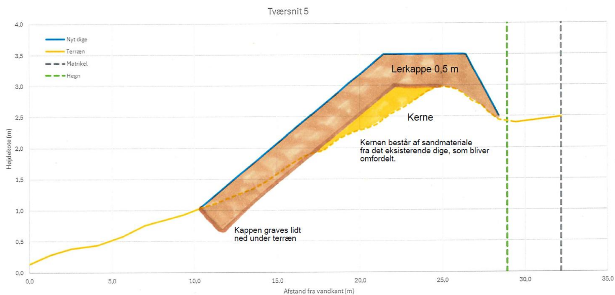
Figur 3 Tværsnit gennem diget. Tværsnittet er placeret ved "TV5" på figur 2.
