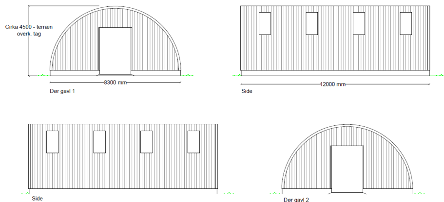
Snittegning som viser det ansøgte projekt.
