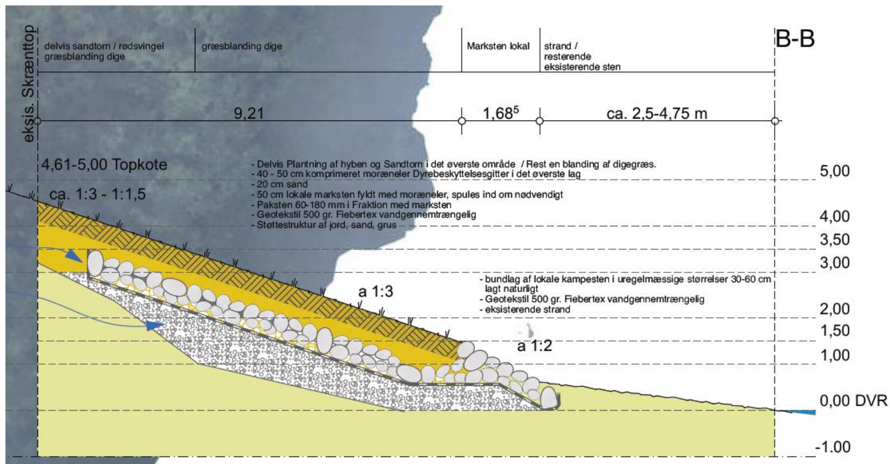
Figur 3.2: Et tværsnit gennem anlægget, fra ansøgningsmaterialet
