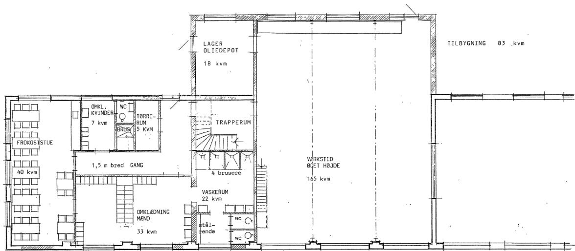
3.ETAPE AF OM-06 TILBYGNING STUEPLAN I MÅL 1:100
