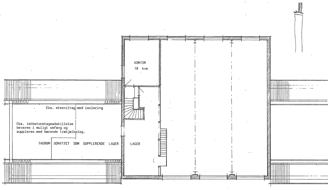
3.ETAPE AF OM-06 TILBYGNING TAGETAGE I MÅL 1:100
